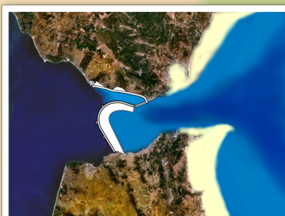
Gibraltár – a fő zárógát és vízerőmű
